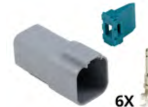
Conector DT04-6P Macho - 6 vias Cód. 1217061
