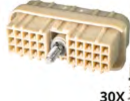
30X Conector do Modulo Fêmea - 30 vias - L/Y Cód. 1204303 TERM: 110022
